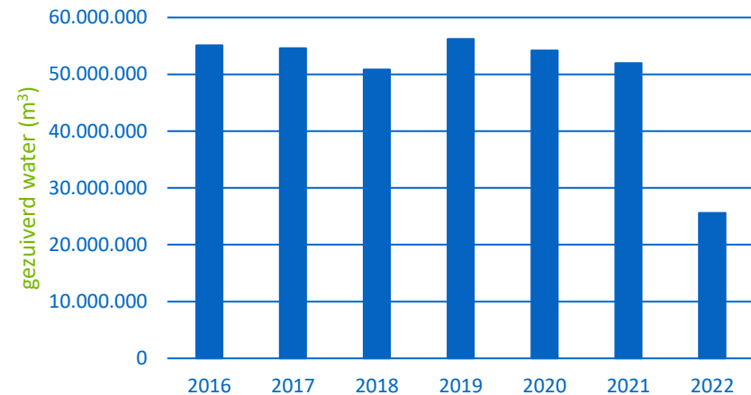
Figuur 2: Hoeveelheid gezuiverd afvalwater t/m juni 2022
